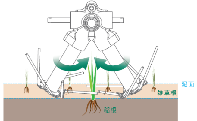
水田除草用回転レーキ、除草の仕組み
